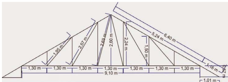
Gambar 5.4. Model Struktur Kuda-Kuda Baja Ringan
