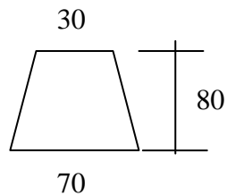
Gambar 5.1. Desain Pondasi Batu Kali
