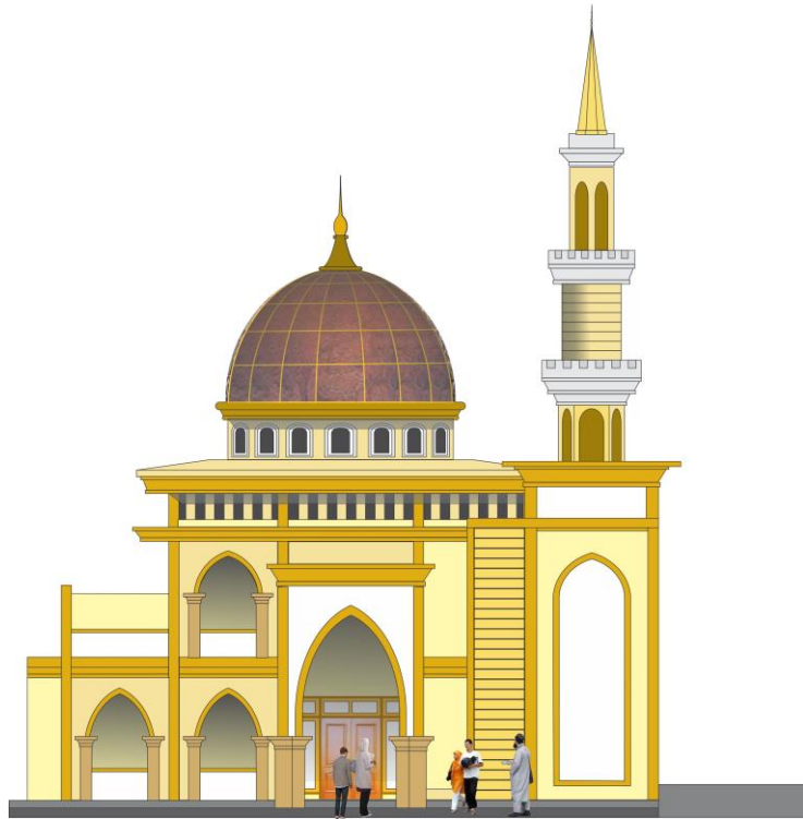
Gambar 5.4. Rencana Desain Tampak Selatan Masjid As Salam
